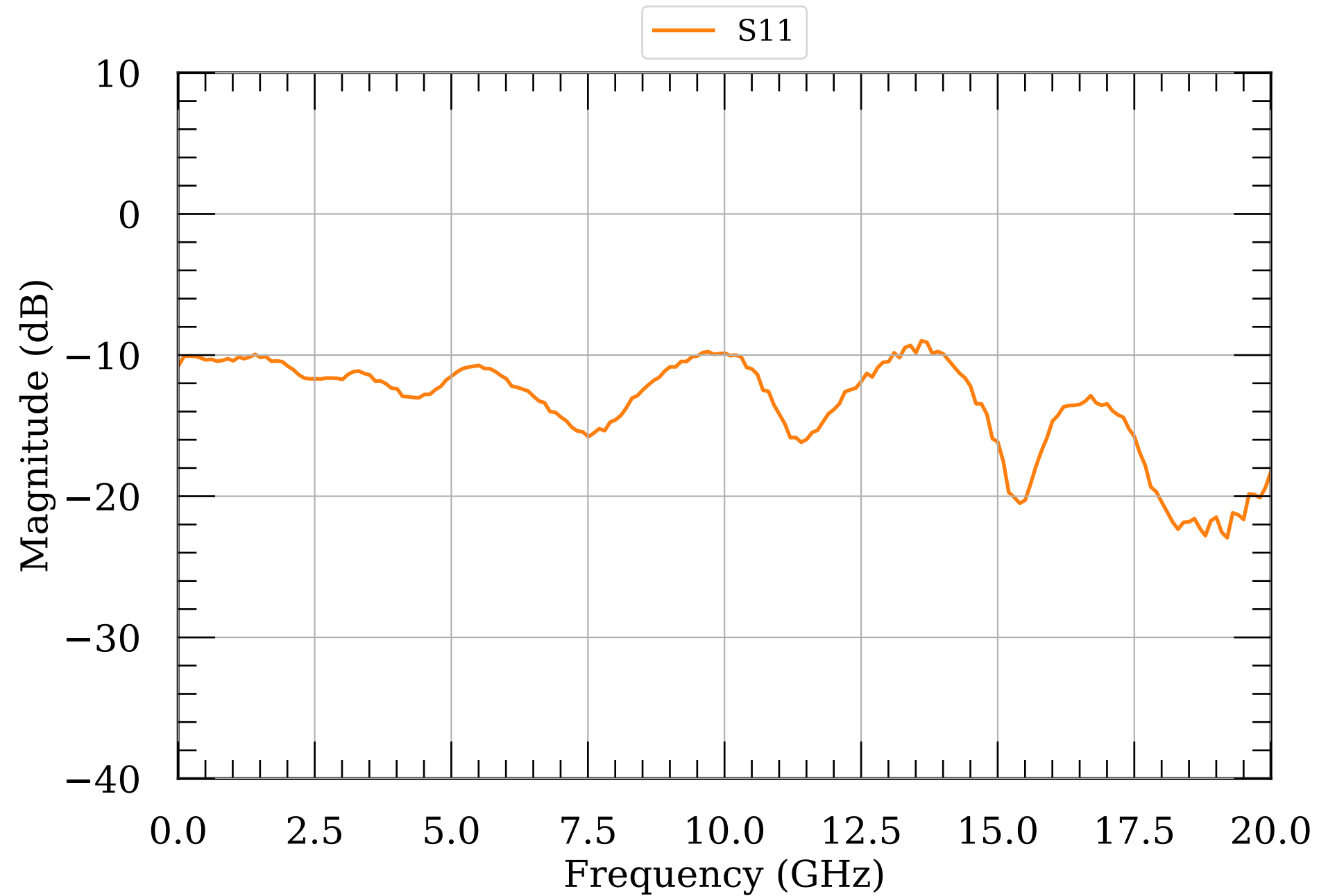
LNA S-params module046v2
